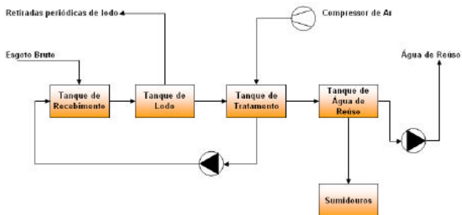
FIGURA: Fluxograma de processo MBR
