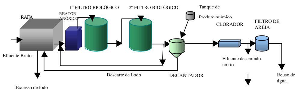
FIGURA: Fluxograma de processo convencional
